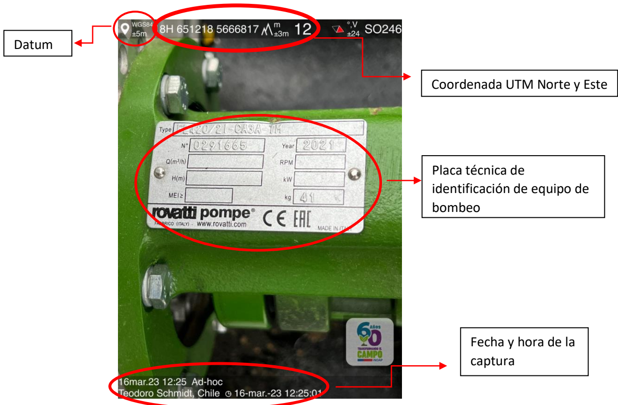
Figura 4. Placa técnica del equipo de bombeo
