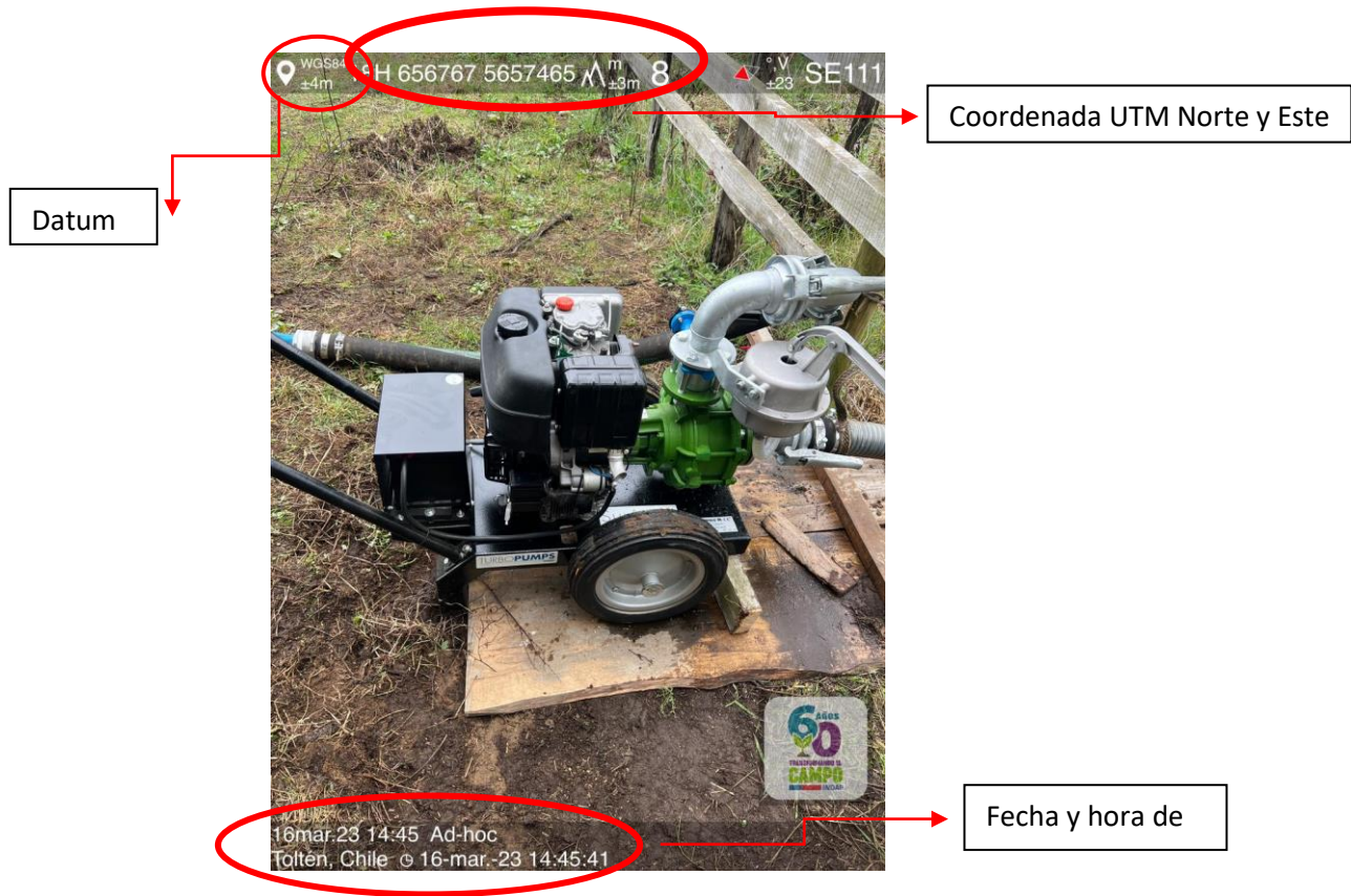
Figura 3. Equipo de bombeo seleccionado realizando la prueba en terreno
